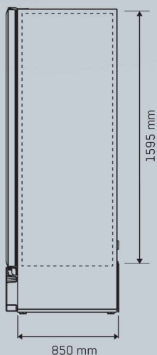
VISTA LATERAL
